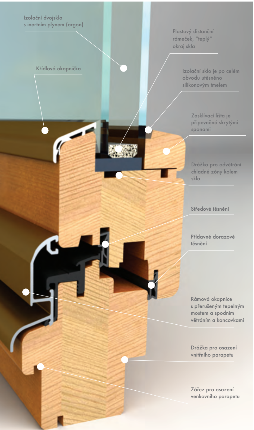
řez oknem
