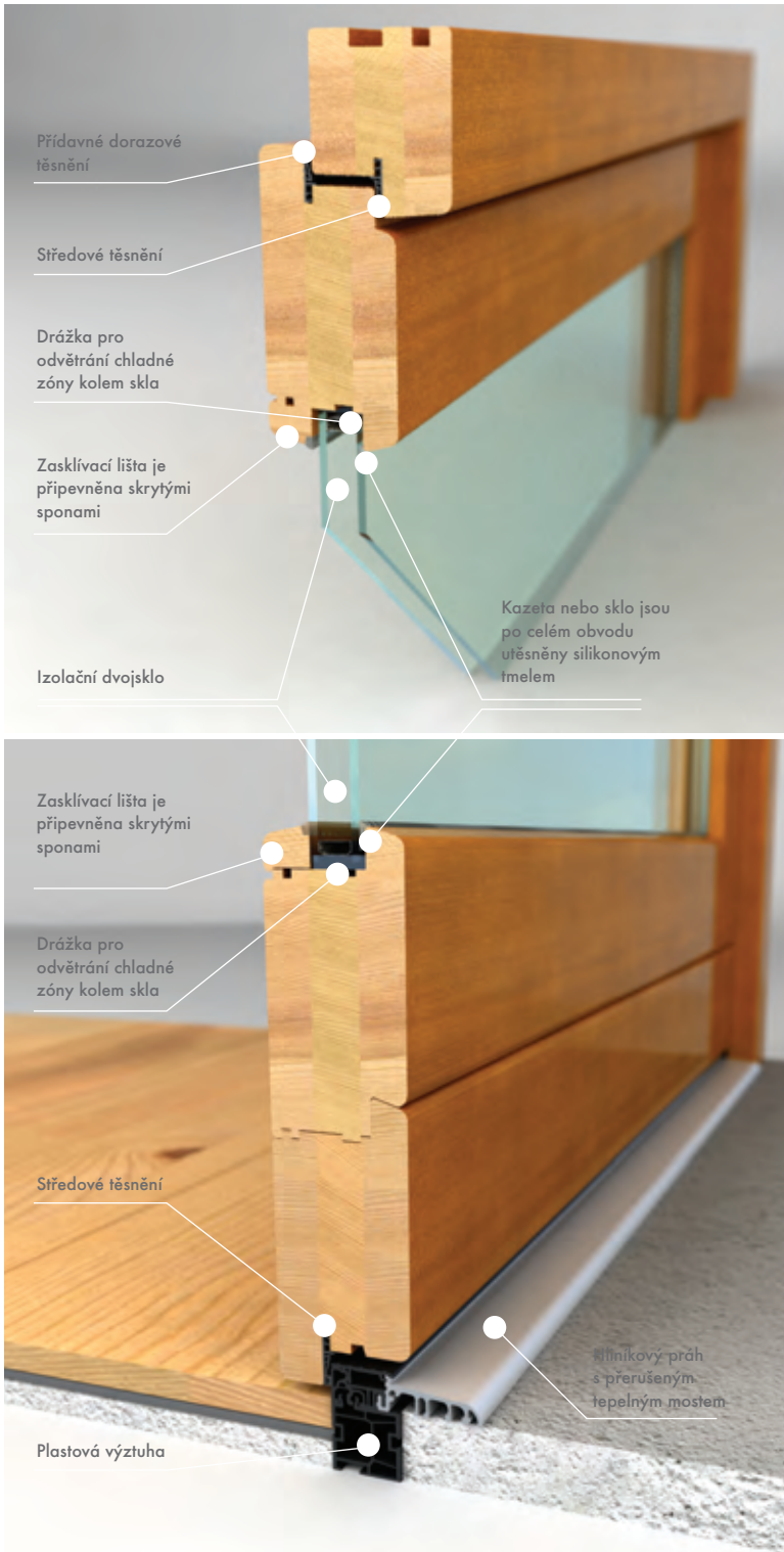
řez dveřmi
